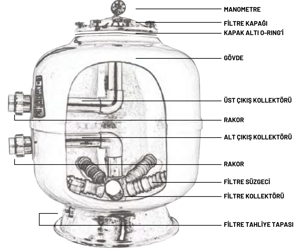
Atlaspool Havuz Filtreleri Yedek Parça Listesi
